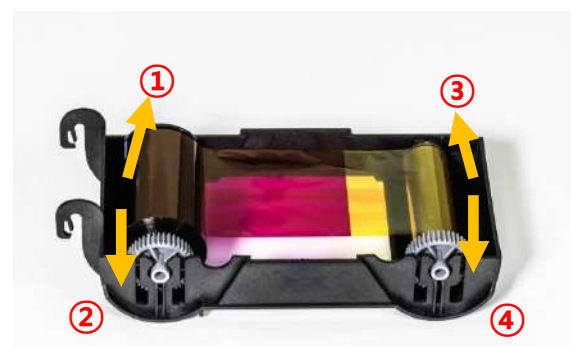
Рис. 16 Загрузка ленты
