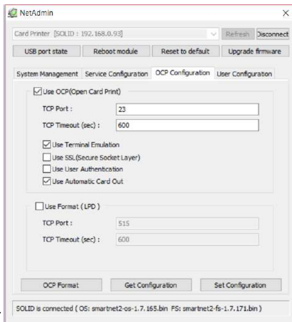
Рис. 87 OCP конфигурирование
