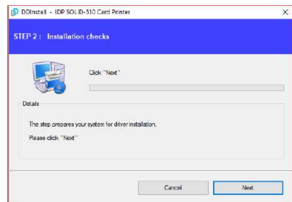
Рис. 39 Установка драйвера
